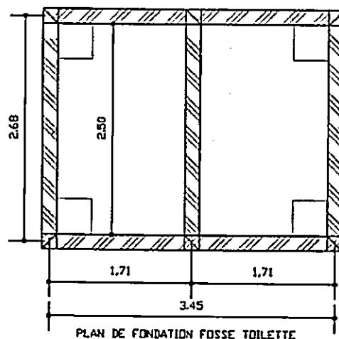
PLAN DE FONDATION FOSSE TOILETTE
